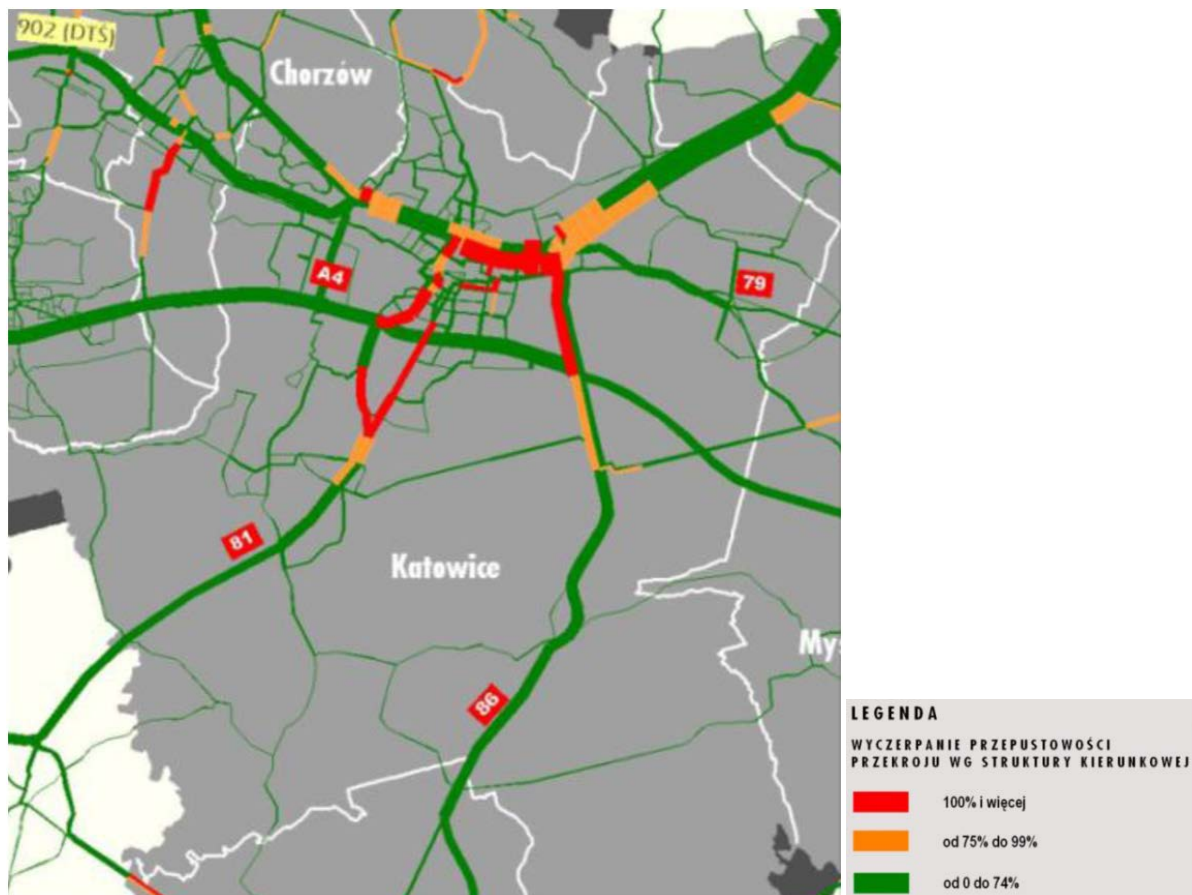
Rys. 1.32. Wyczerpanie przepustowości układu drogowego Metropolii "Silesia" – fragment sieci Katowic, stan na 2008
